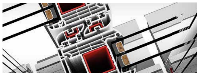
Im Standard: drei Riegelhaken zur Erhöhung der Sicherheit. Möglichkeit des Einbaus von modernem Sicherheitszubehör zur Verbesserung des Einbruchsschutzes.
